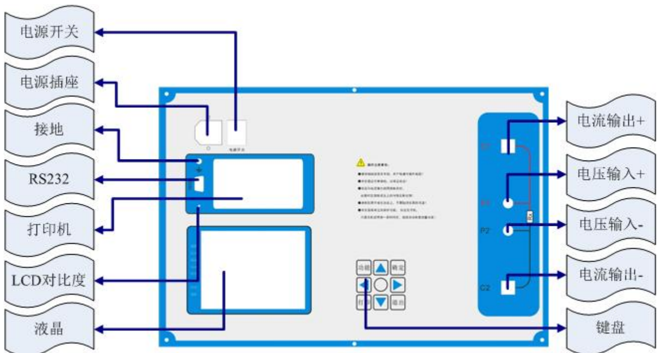
图 2 面板结构图
