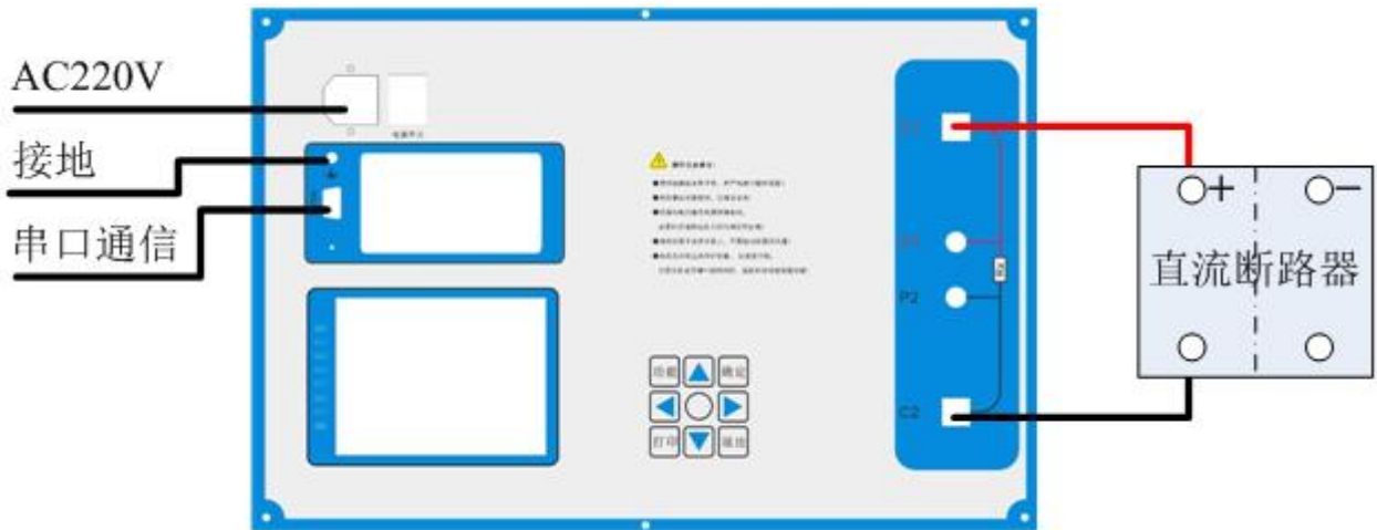
图 1 接线示意图
