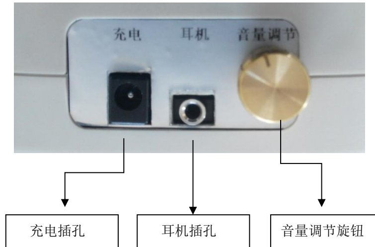
主机底面图
