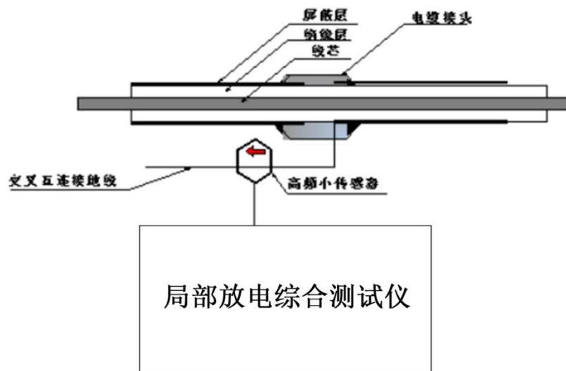
电缆接头局放在线现场连接示意图
