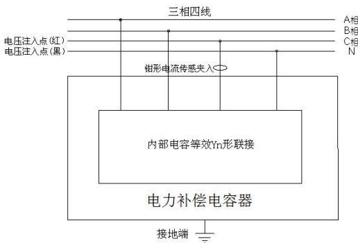
C 相接线
