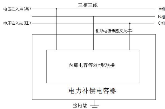
C 相接线
