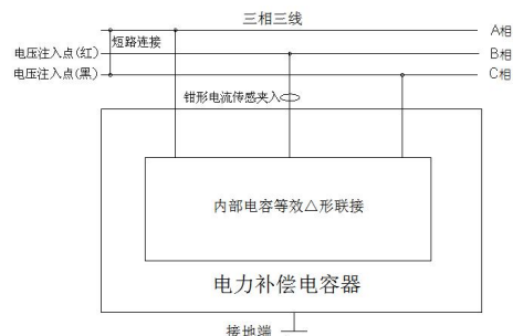
B 相接线
