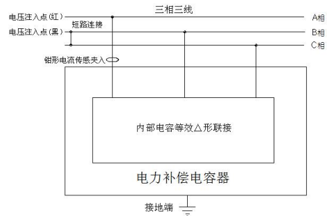
A 相接线
