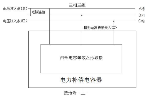
C 相接线
