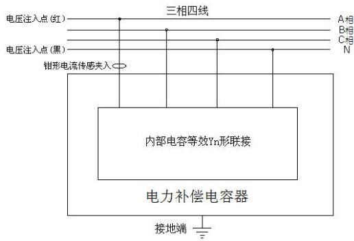
A 相接线
