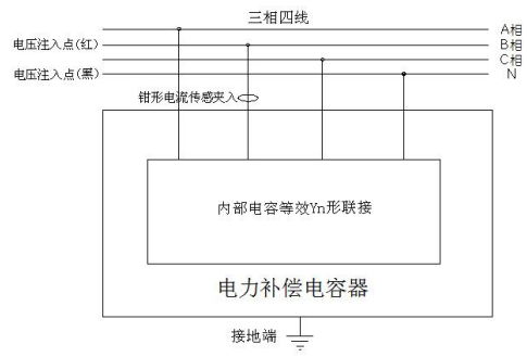
B 相接线
