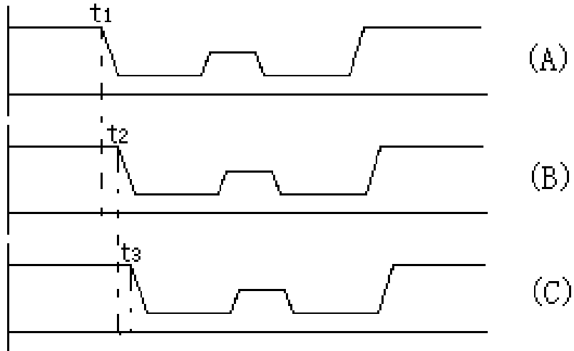
不同期的三相波形（假设 A 相超前 B 相，B 相超前 C 相）
